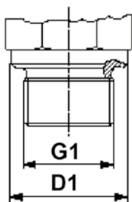
DIN3852-2 形式B IS01179-4 硬密封结构
