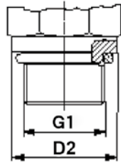
UN/UNF-2A O型密封圈 ISO 11926-2. 3.
