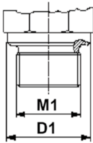
DIN3852-1 形式B ISO1179-4 硬密封结构
