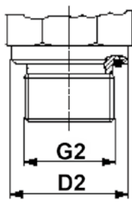
DIN3852-11 形式E IS01179-1 带弹性体密封结构
